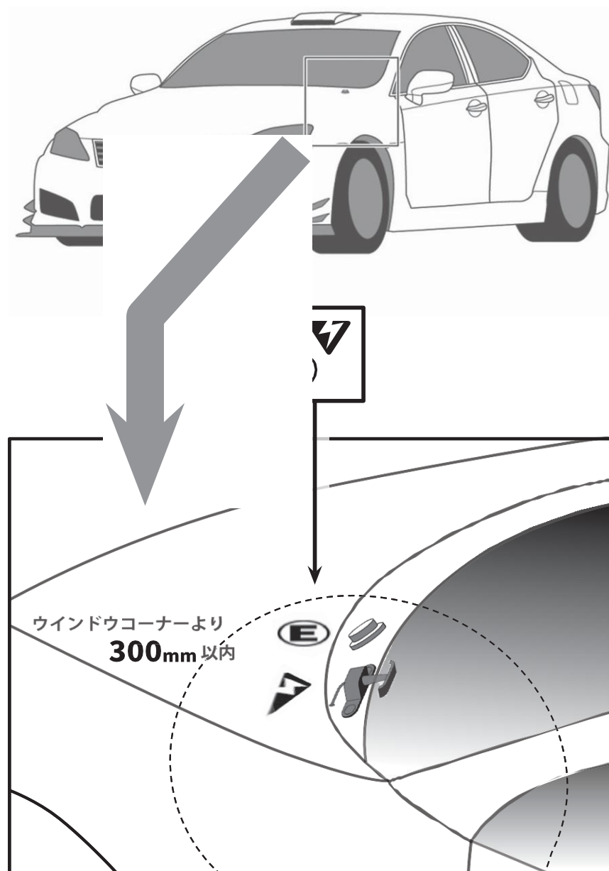
（図 13-1）マスタースイッチおよびカットオフスイッチ取付場所
